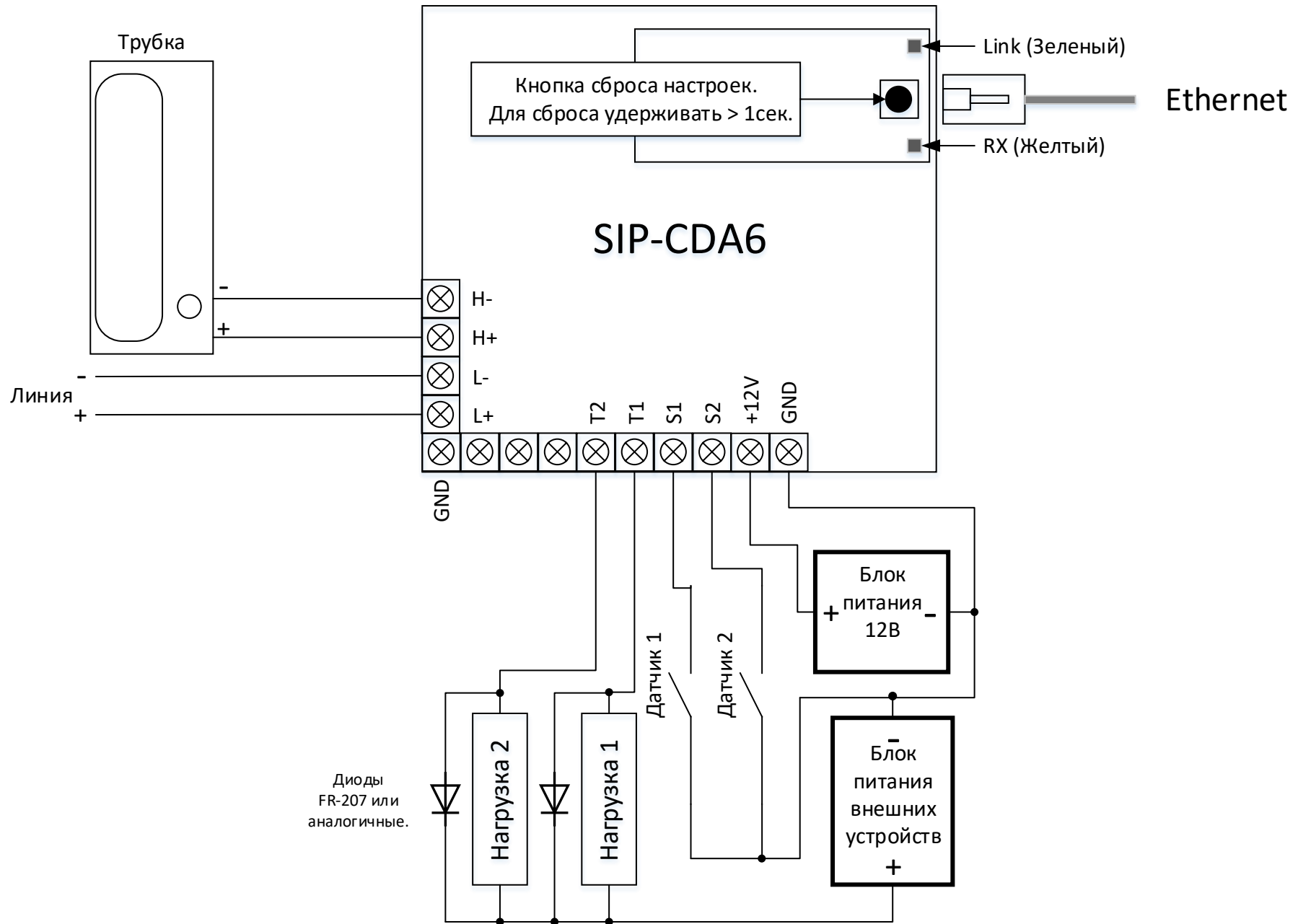
Схема подключения SIP-CDA6 к линии трубки.
