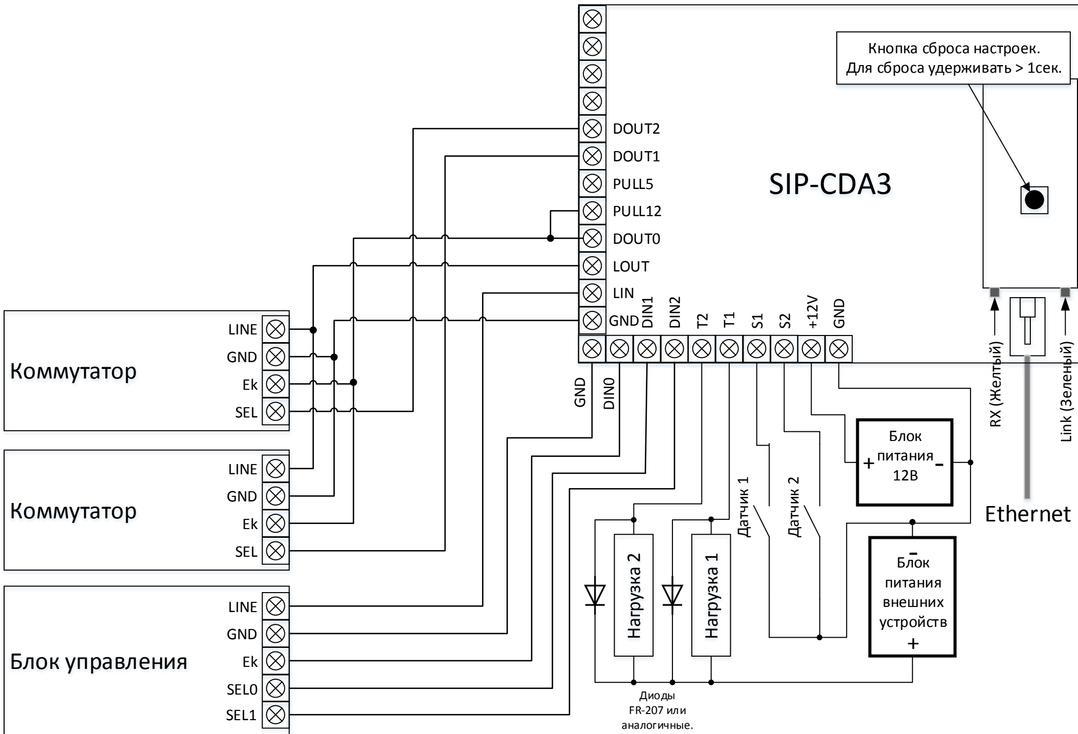
Схема подключения SIP-CDA3 к домофонам Визит.
