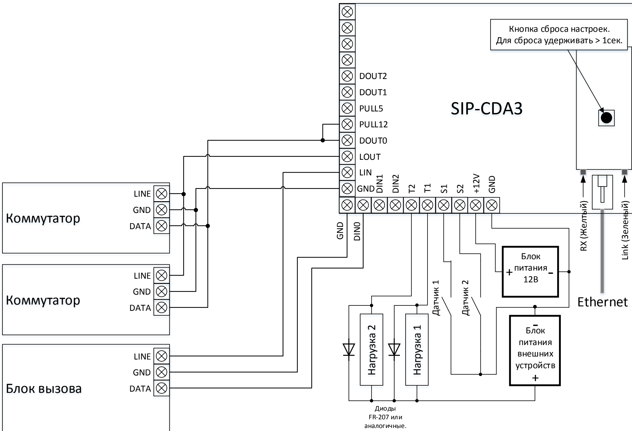
Схема подключения SIP-CDA3 к домофонам Метаком.
