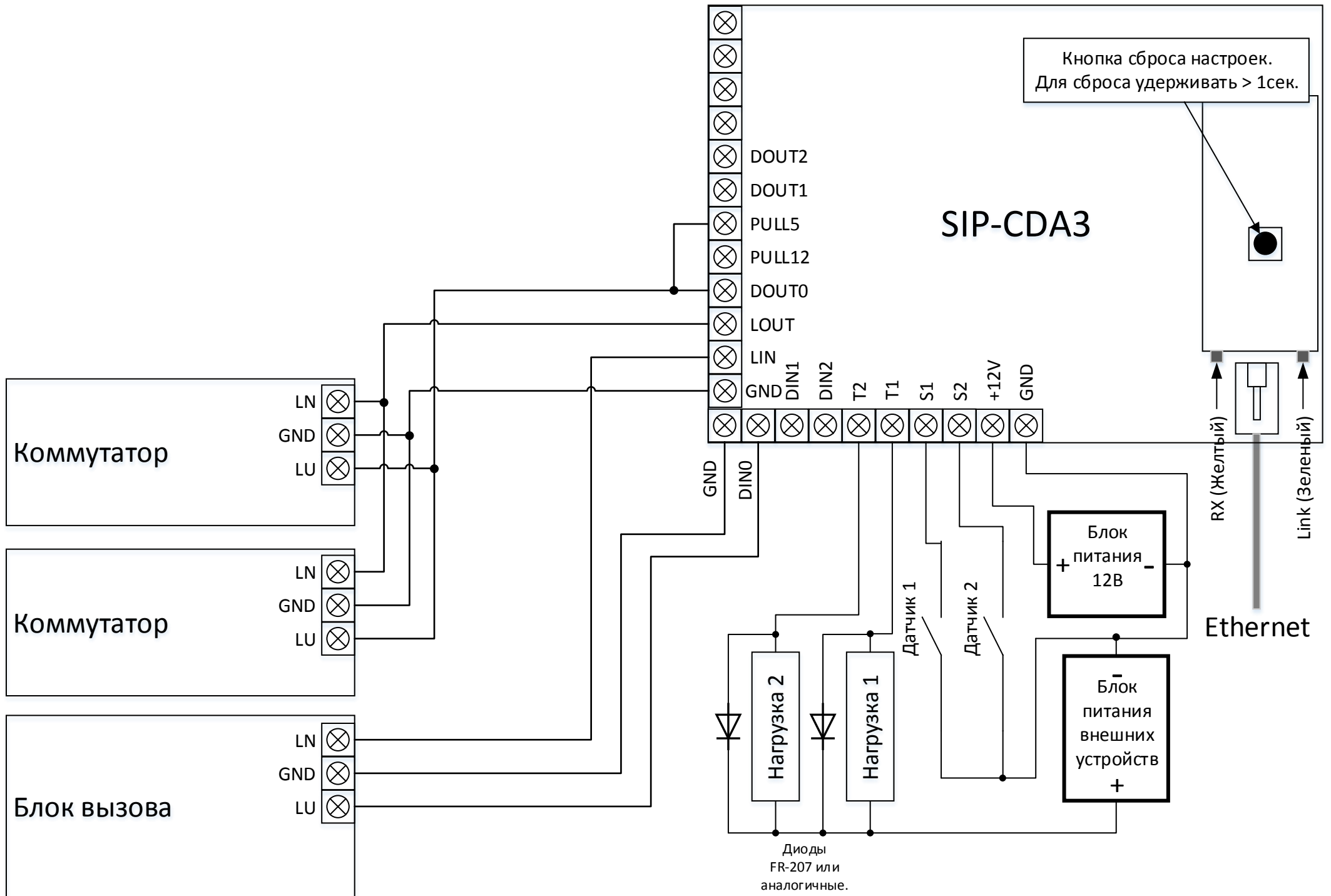
Схема подключения SIP-CDA3 к домофонам Элвис.
