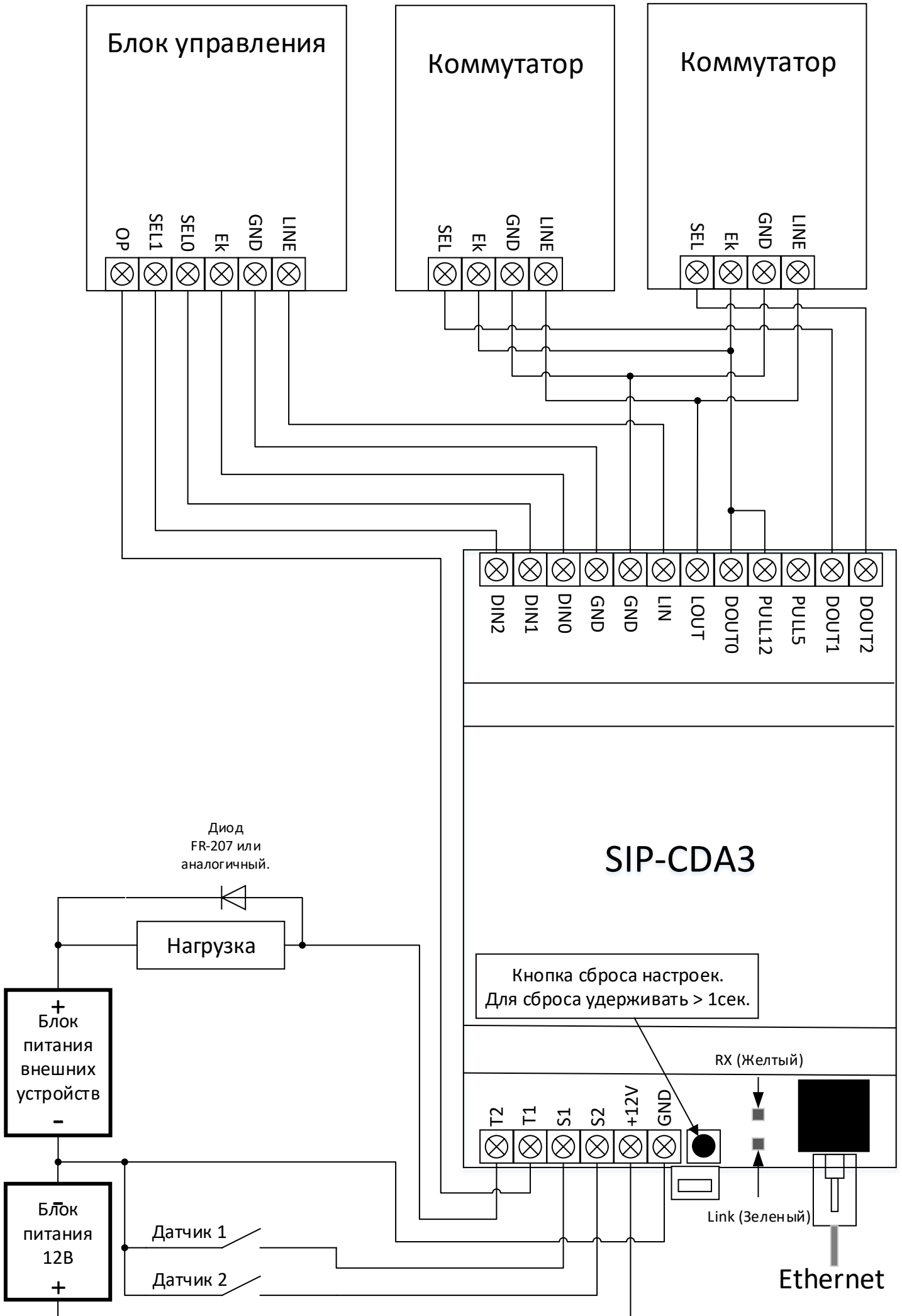
Схема подключения SIP-CDA3 к домофонам Визит.
