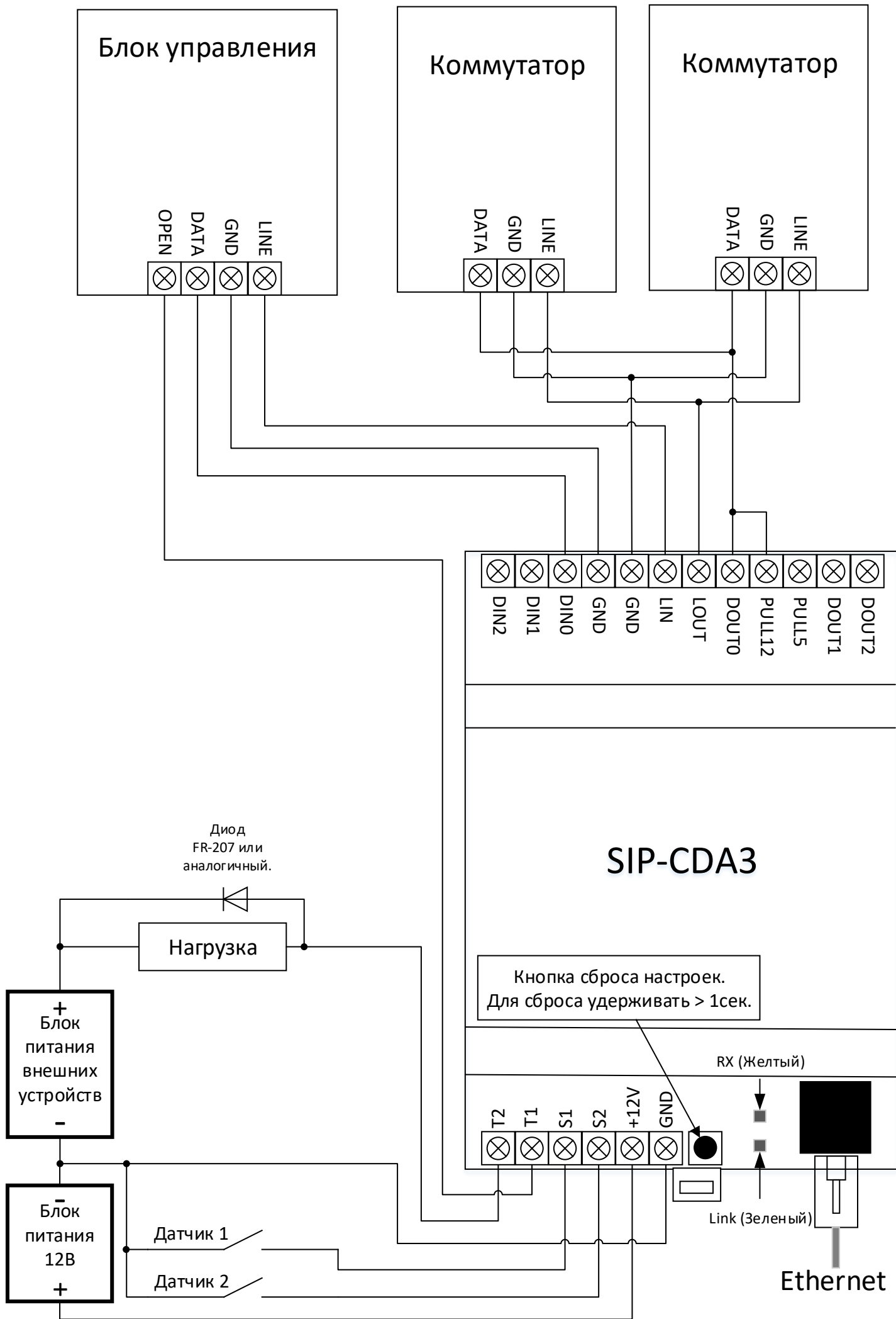
Схема подключения SIP-CDA3 к домофонам Метаком.
