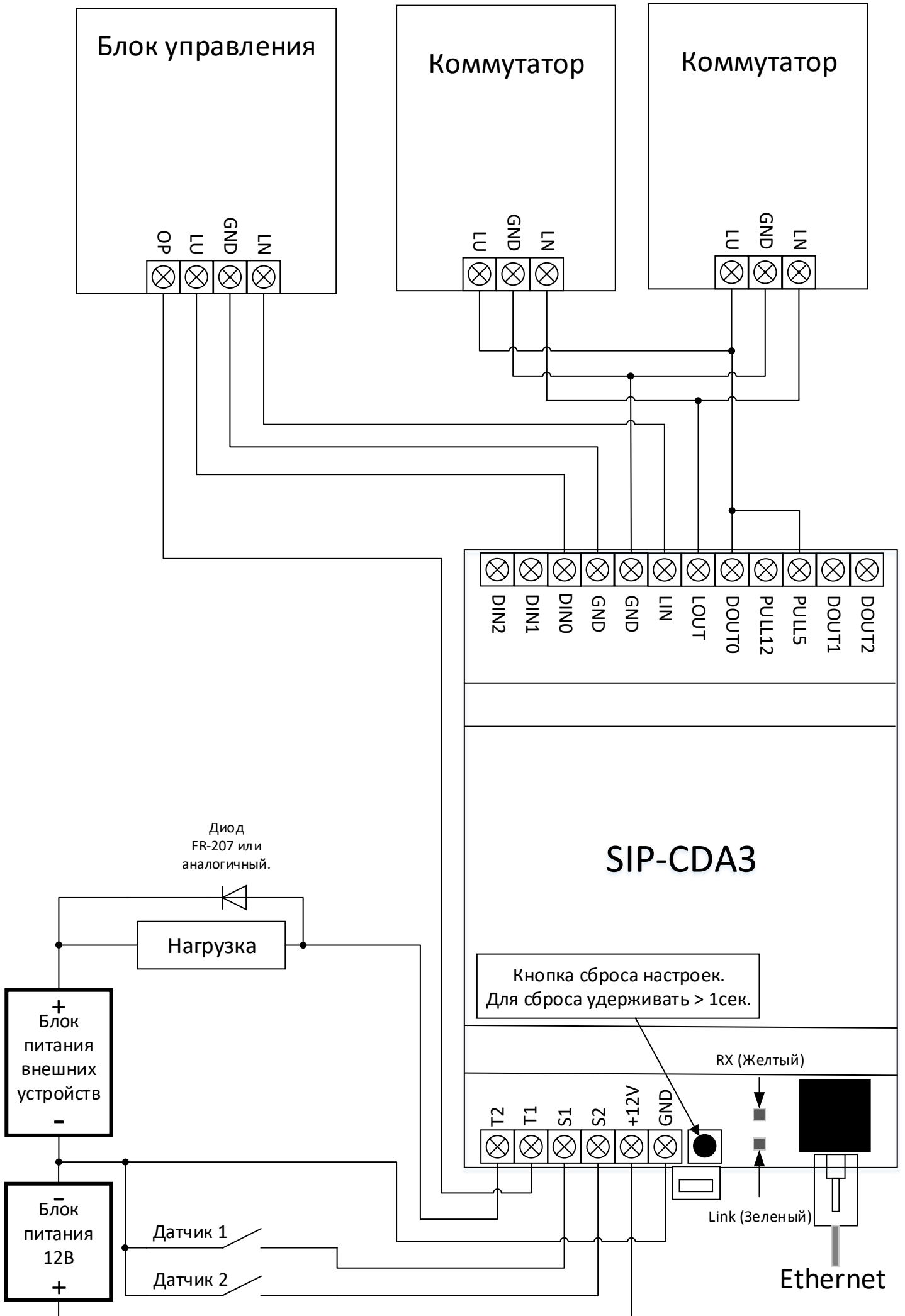
Схема подключения SIP-CDA3 к домофонам Элтис.
