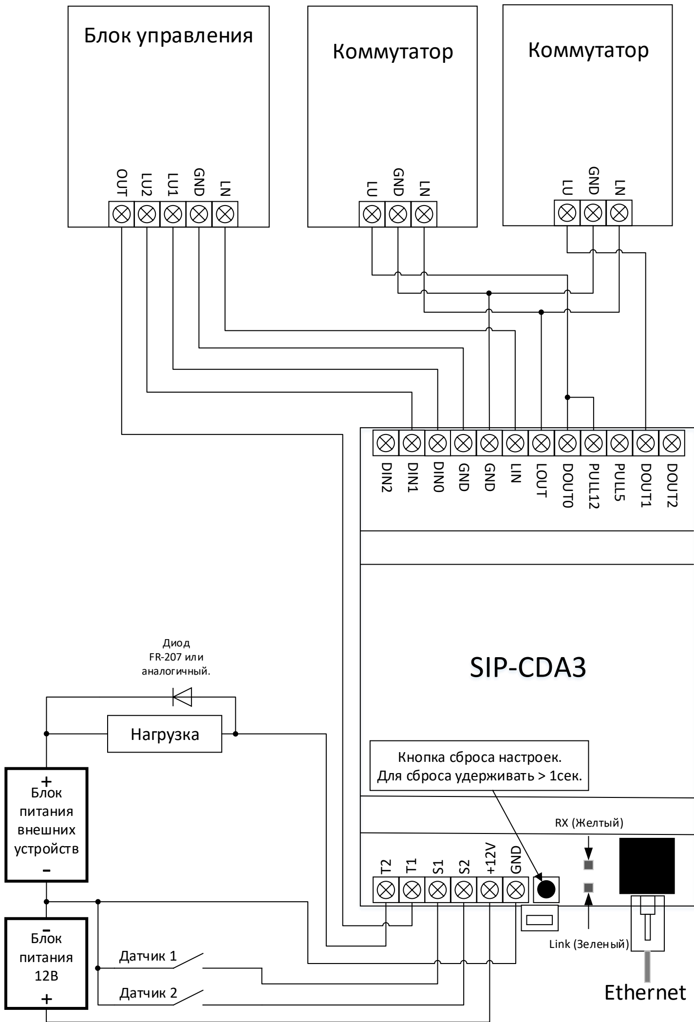
Схема подключения SIP-CDA3 к домофонам Цифрал.
